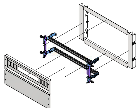
PANNELLO TIPO CHIUSO DA 538X149 MM
